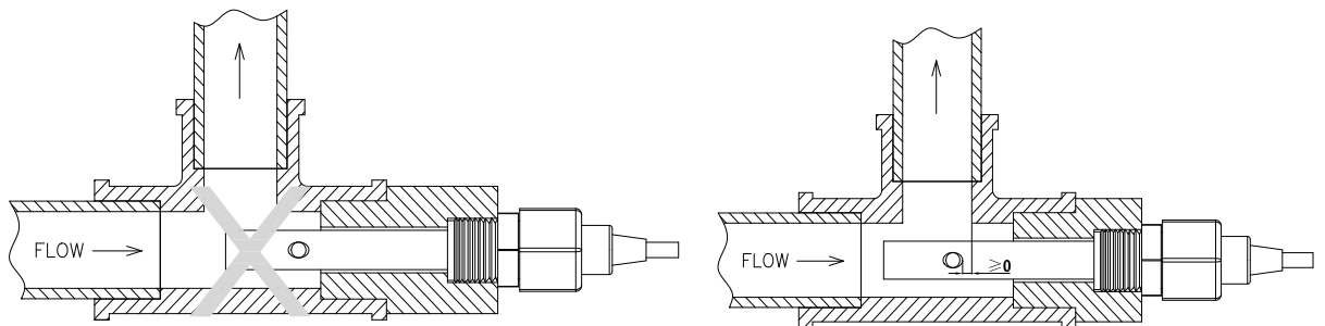
图 A 错误安装方式
